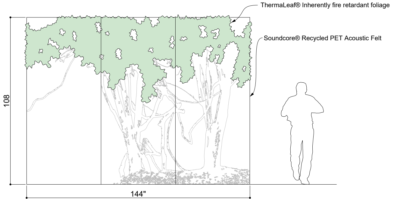
① ELEVATION 1
